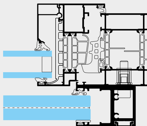
Soleal Next 75: fissaggio dall'esterno
